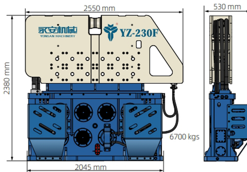
Вибропогружатель Yongan YZ 230F
